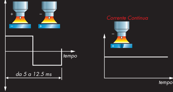
Corrente Alternata ad Onda Quadra
